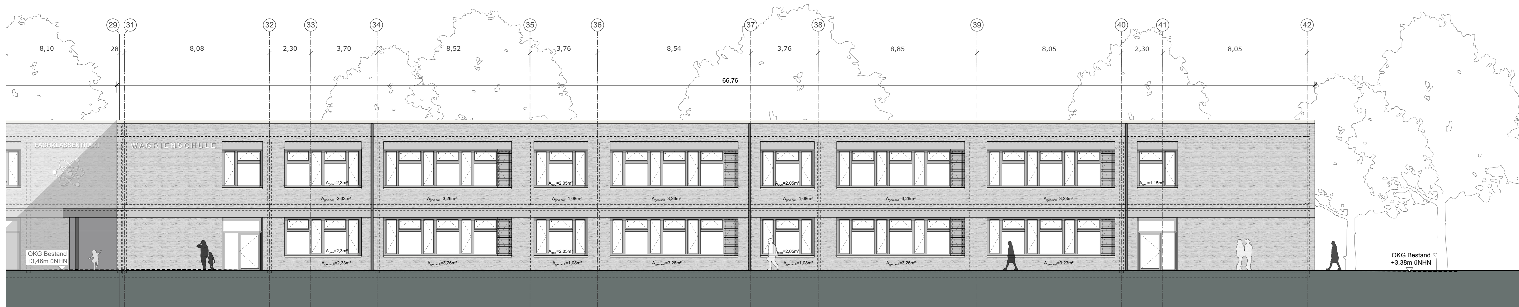
Gemeinschaftsschule Ansicht West, M 1:100
