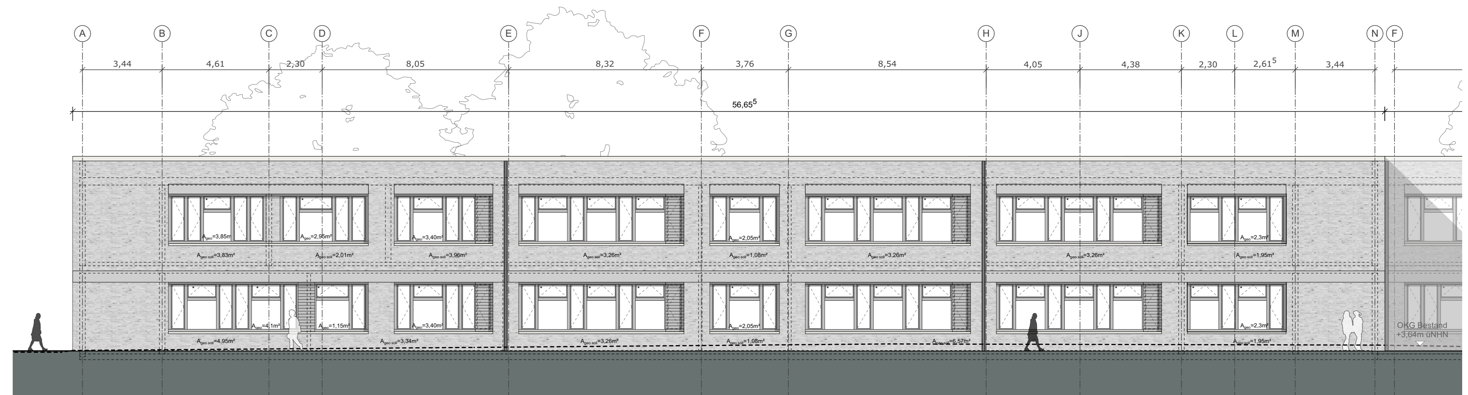
Gemeinschaftsschule Ansicht Süd, M 1:100
